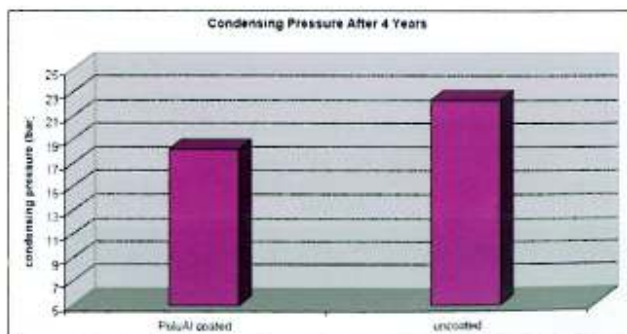
FIG. 11 Pressione di condensazione dopo 4 anni.
