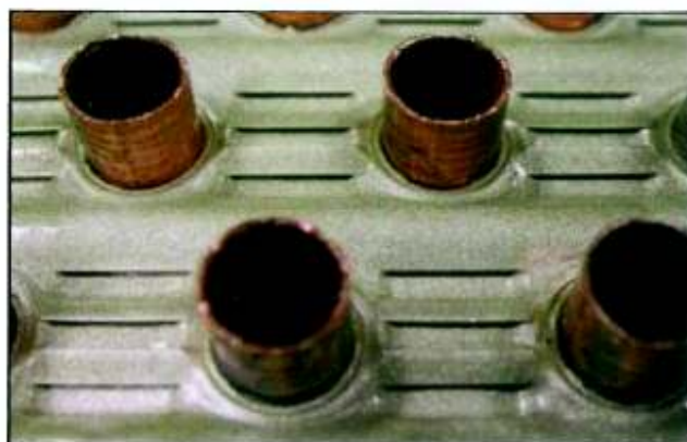
FIG. 6 Aletta turbolenzata rivestita.
