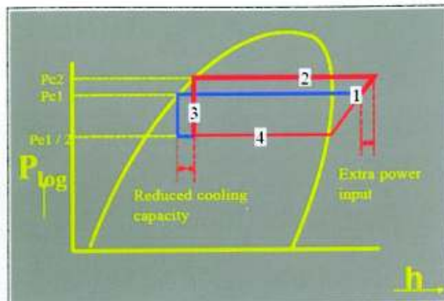
FIG. 2 Effetto della corrosione su consumo energetico.
