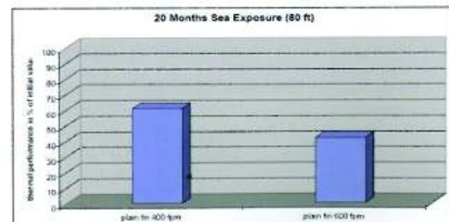
FIG. 4 Esposizione per 20 mesi a ca. 25 metri dal mare.
