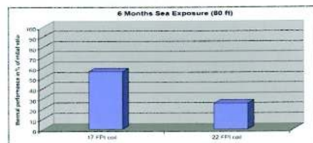
FIG. 3 Esposizione per 6 mesi a ca. 25 metri dal mare.
