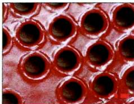
Fig. 21-22 Applicazione interno tubi. Application inside the tubes.
